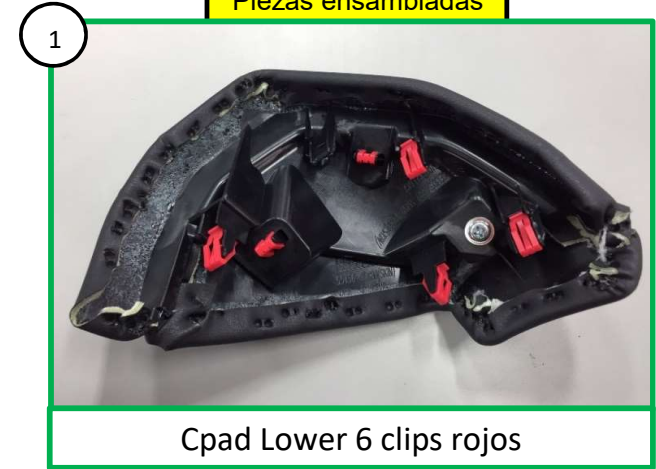
Piezas ensambladas
