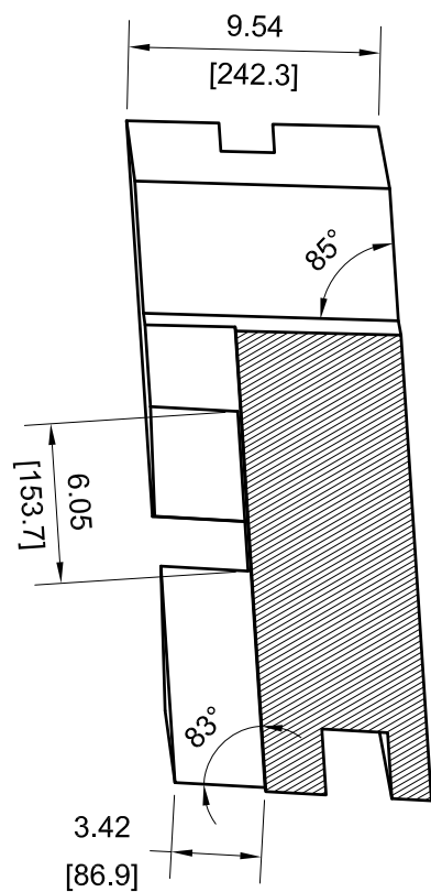
SECTION VIEW D2-80
